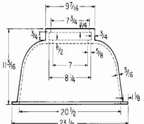
6860 160 Base
